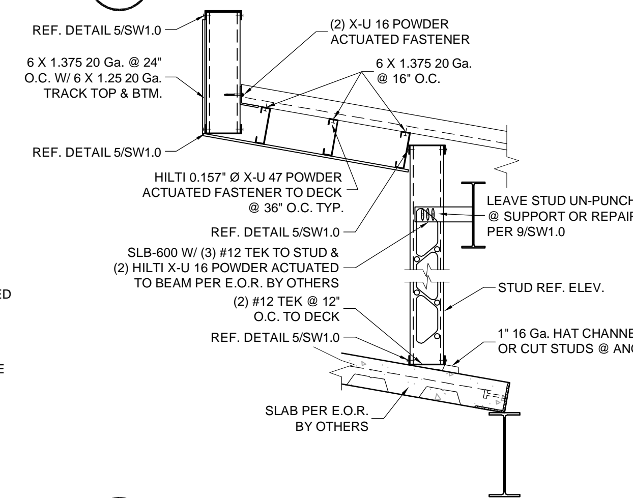
15 WALL ON ROOF N.T.S.
