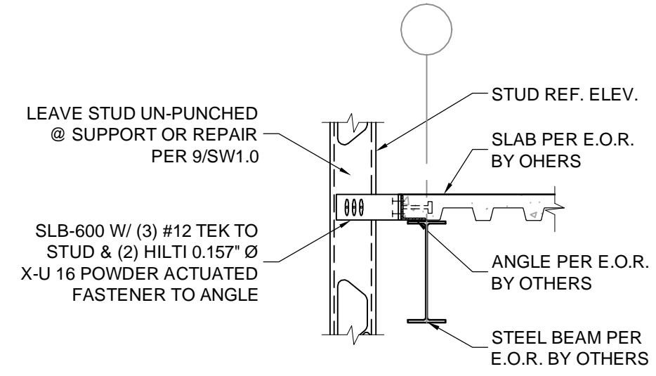
7 WALL TO FLOOR N.T.S.
