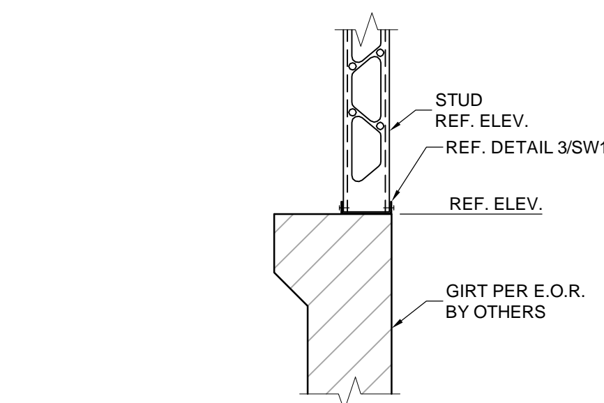
17 WALL TO GIRT N.T.S.
