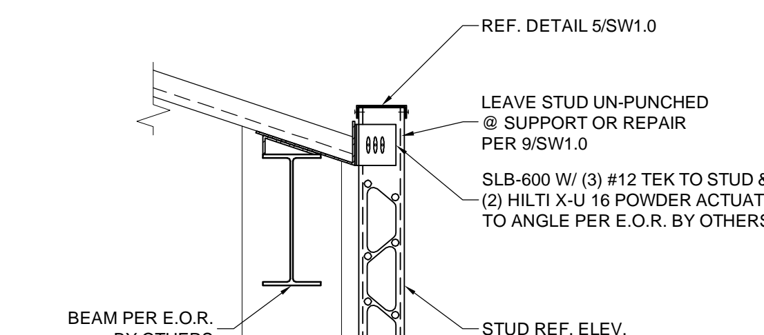
15 WALL ON ROOF N.T.S.
