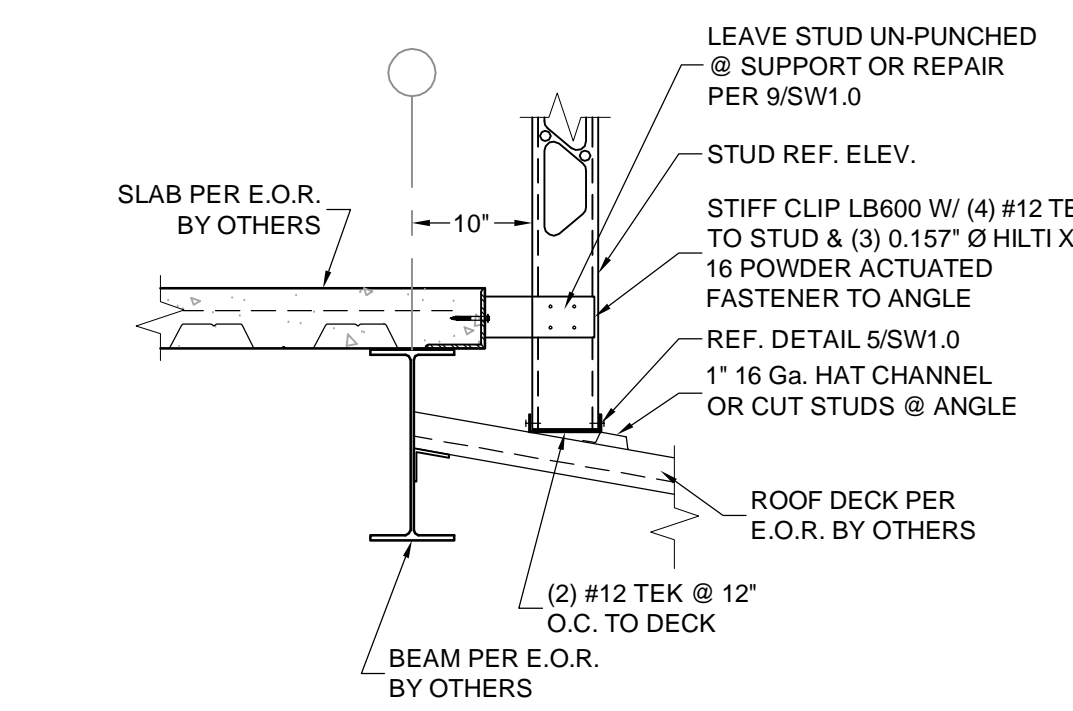
18 STUD TO DECK N.T.S.
