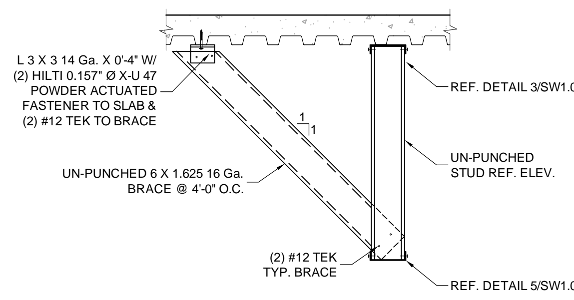
6 WALL W/ BRACE N.T.S.
