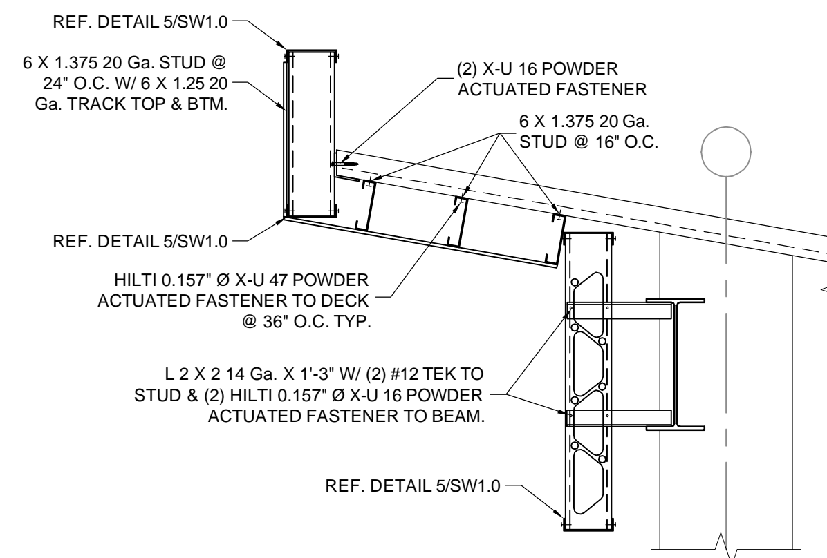
9 HIGH EAVE N.T.S. 8/S-403
