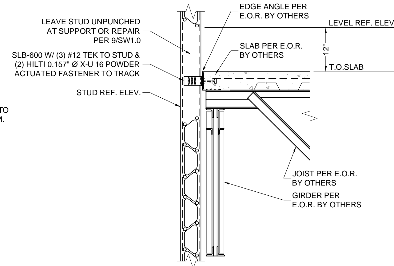
3 WALL @ GIRDER N.T.S. 7/S-405
